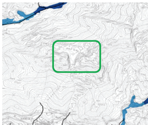
Fig. 5 - Estratto della Tavola 20 B – Planimetria della pericolosità idraulica del Comune di Carrara. Nel riquadro l'area di specifico interesse.
